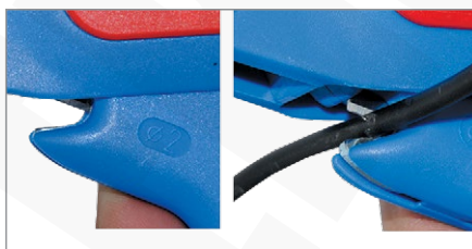
Odcięcie przewodu
