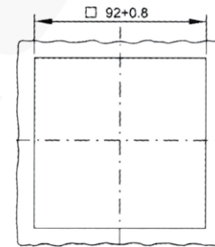
Otwór instalacyjny
